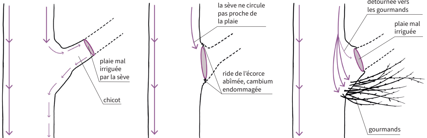
Schéma 9 : Mauvaise coupe chicot trop loin du tronc
